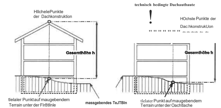
Figur 4.1.a Gesamthöhe
