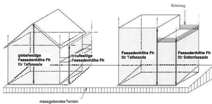
Figur 4.2.a Fassadenhöhe
