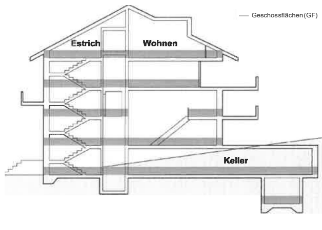
Figur 7.2 Geschossflächenziffer
