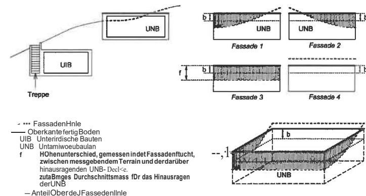
Figur 1.3 und 1.4 Unterirdische Bauten, Unterniveaubauten
