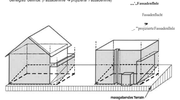
Figur 2.2.b Fassadenflucht und Fassadenlinie (in geneigtem Gelände)
