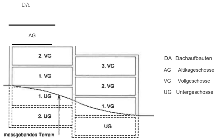
Figur 5.1 Geschosse und Geschosszahl
